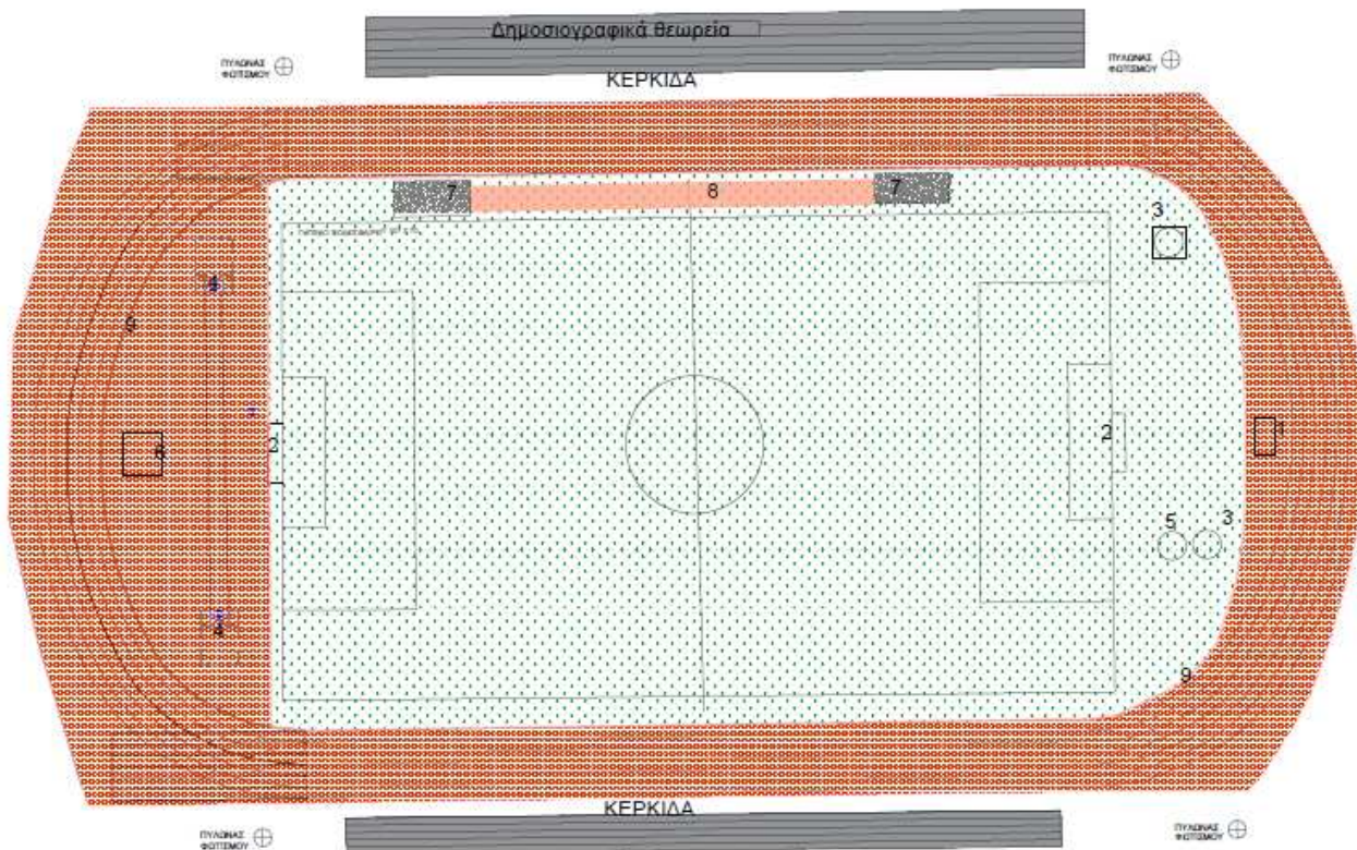
Εικόνα 1 ΓΕΝΙΚΗ ΔΙΑΤΑΞΗ ΕΓΚΑΤΑΣΤΑΣΗΣ
