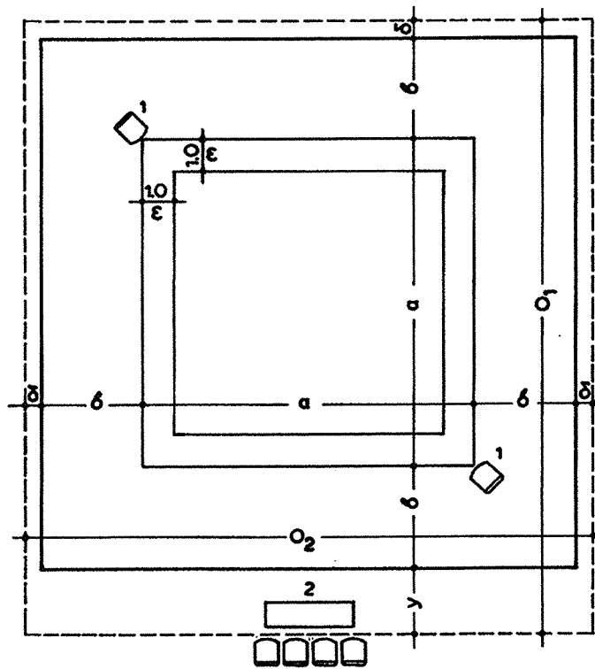
ΚΑΤΩΗ ΑΓΟΝΙΣΤΙΚΟΥ ΧΩΡΟΥ ΚΛ.1:200
