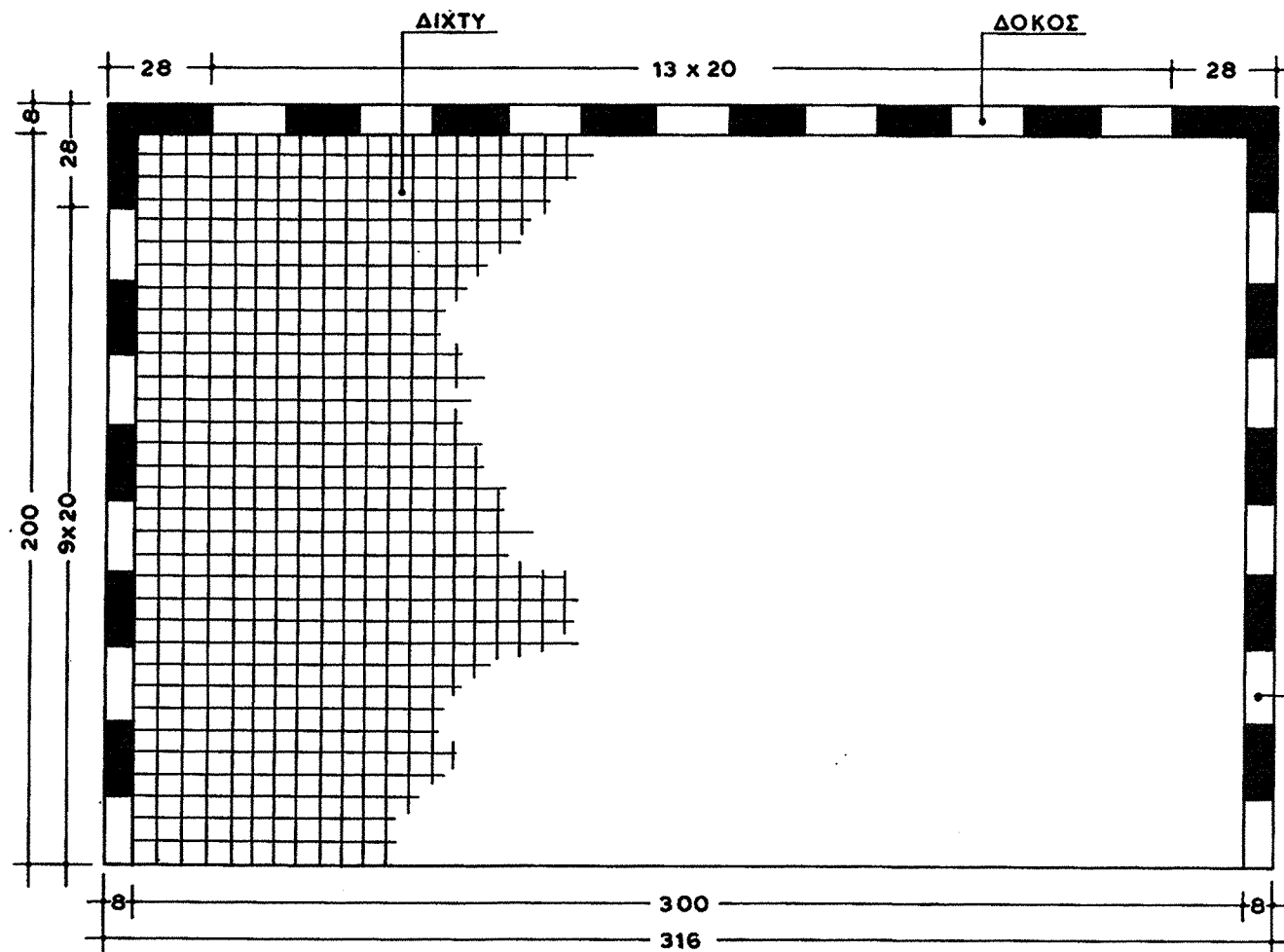
ΟΨΗ ΚΛ.1:20
