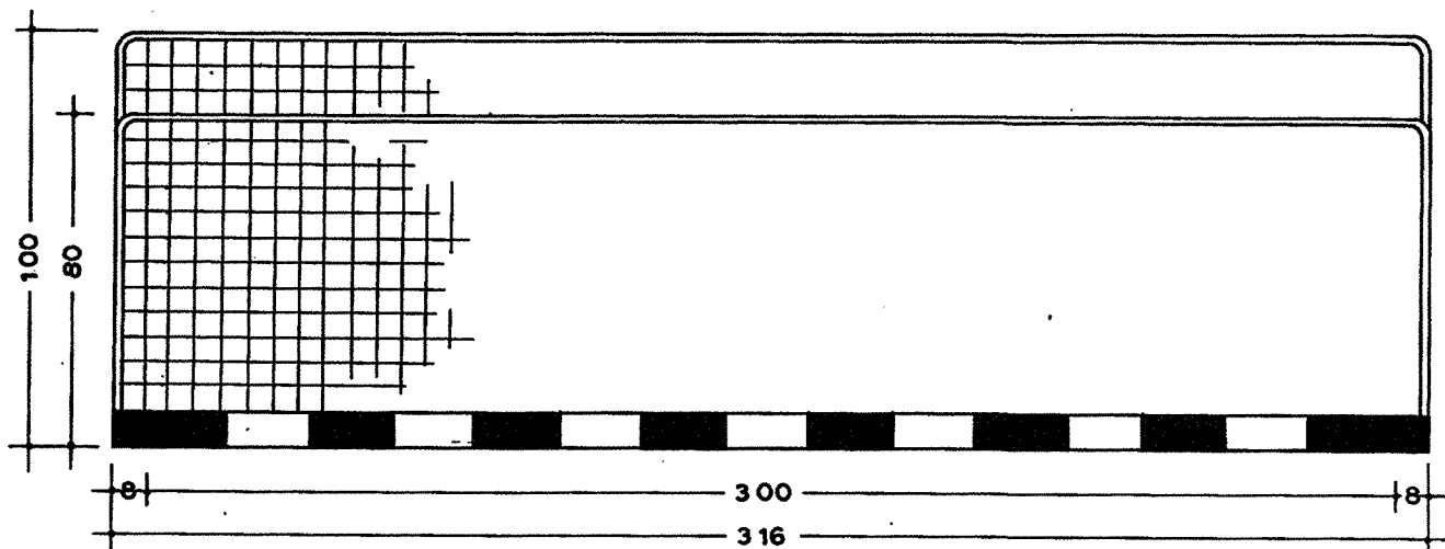
ΚΑΤΩΗ ΚΛ.1:20
